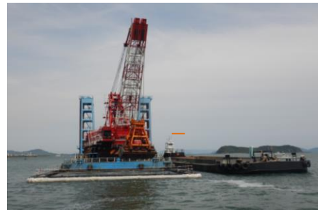
Grab 浚渫船
