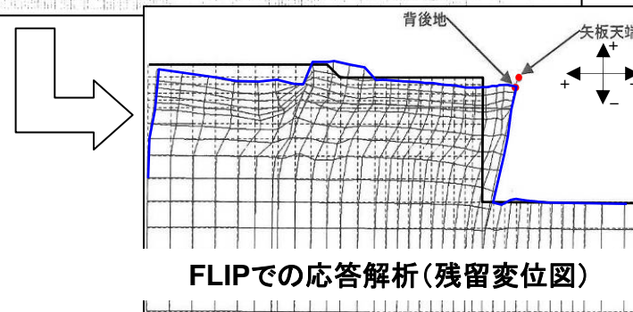
図-1 チャート式診断システムとFLIP解析の比較(水平変位量)
