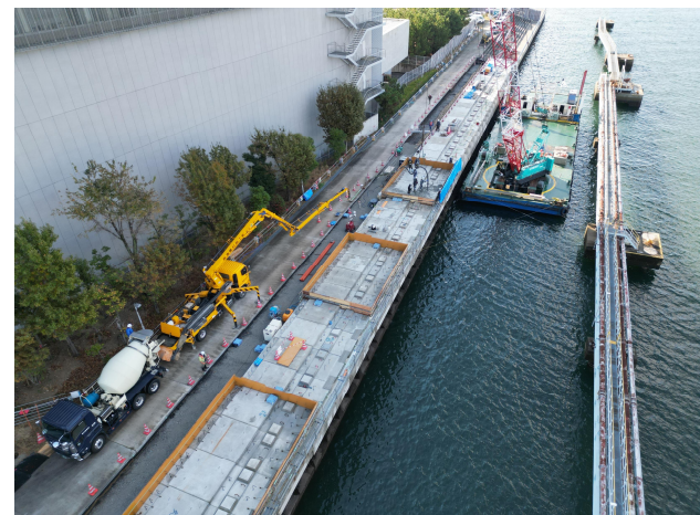
⑥ 上部コンクリート打設
