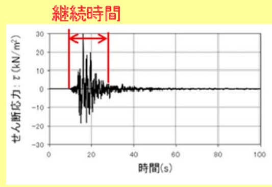
地震動の継続時間が短い波形 (阪神大震災)
